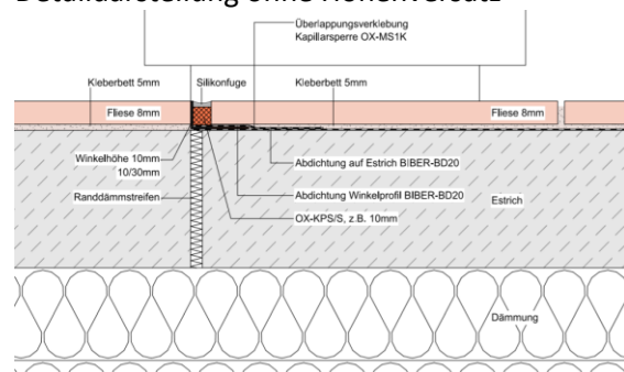
Detaildarstellung ohne Höhenversatz
